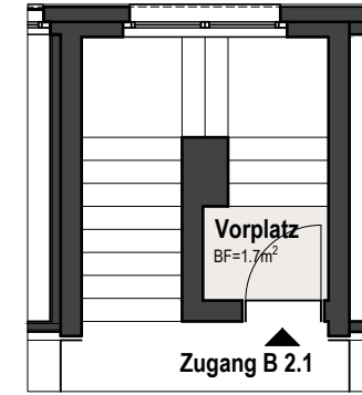
Zugang 1. Obergeschoss
